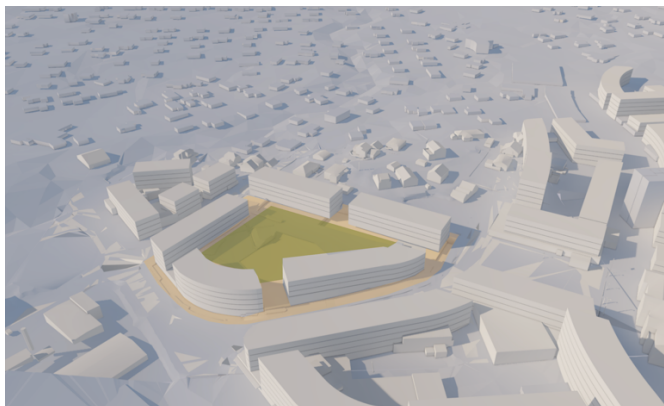
Maks utnyttelse av S11 ihht sentrumsplanen hvis all BRA over 1. etasje benyttes som bolig
