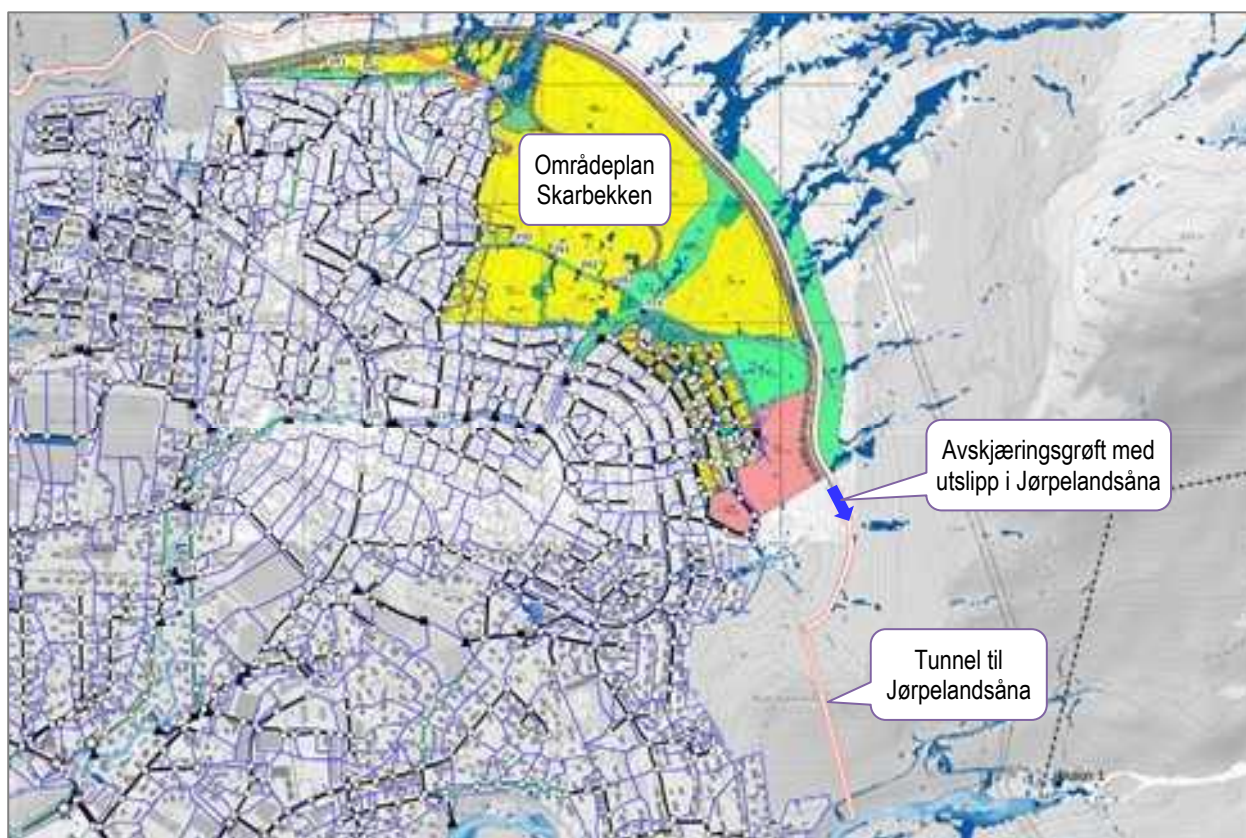
Figur 9.53 Avskjæringsgrøft nordøst for Jørpeland, fra Klovsteinsbekken langs planlagt vei til Fullshammaren, og flomtunnel gjennom fjellet med utslipp i Jørpeldandsåna (vann-dybde scenario A 2.2).
