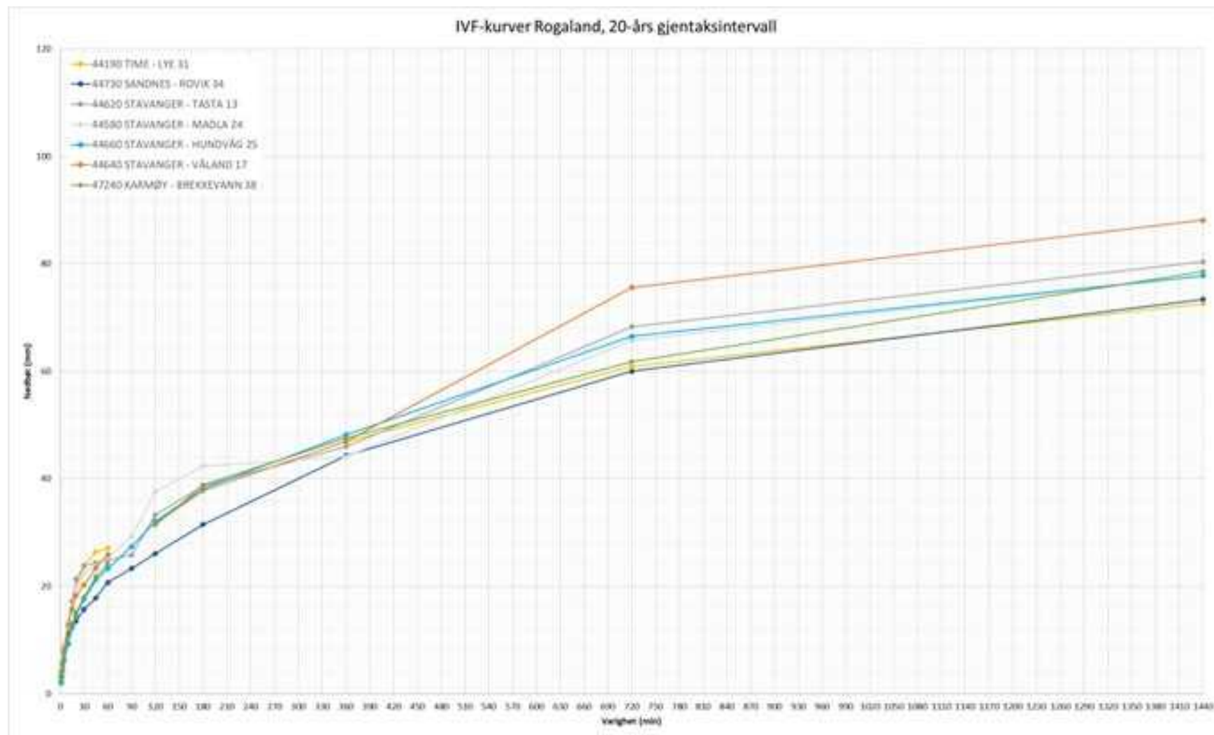
Figur 3 IVF-kurver fra nedbørstasjoner i nærheten av Strand kommune for 20-års gjentaksintervall opptil 24 timer varighet; antall sesonger er angitt etter serienes navn. Kilde: Klimaservicesenter.no, lastet ned 05.06.2020.
