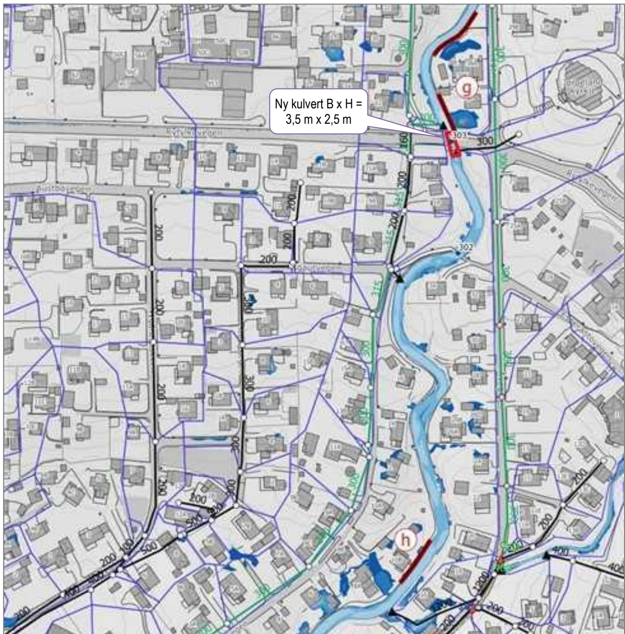
Figur 9.28 Sikring mot 200-års overvannsflom på sted g og h sentralt i Jørpeland (vanndybde scenario A 2.2).
