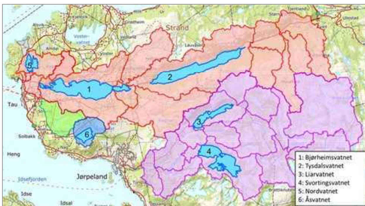
Figur 5.2 Innsjøer tatt med i nedbør-avløps-modellen som magasiner i de fire simulerte nedbørfeltene Taelva (rød), Strandåna (grønn), Fjellsåna (blå) og Jørpelandsåna (fiolett).
