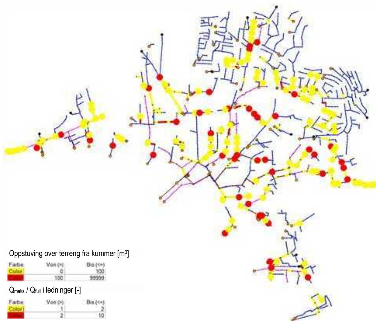
Figur 9.3 Resultater fra koblet ledningsnettberegning Jørpeland scenario A 2.2 (200-års overvannsflom, 60 minutters varighet): Kummer med oppstuvning over terreng og fulle ledninger.
