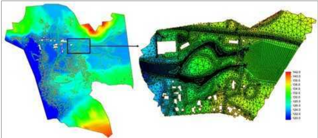
Figur 5.3 Hydraulisk modell for delområdet Tau med utklipp av beregningsnettets rundt utløpet av Bjørheimsvatnet. Fargeskalaen viser terrenghøyder i moh +100 m.
