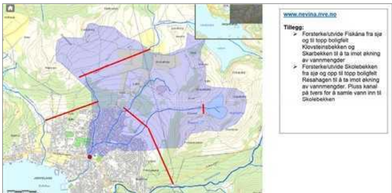
Figur 9.50 Strand kommunes forslag for plassering av avskjæringsgrøfter og en dam ovenfor Jørpeland. Kilde: J. Leland.
