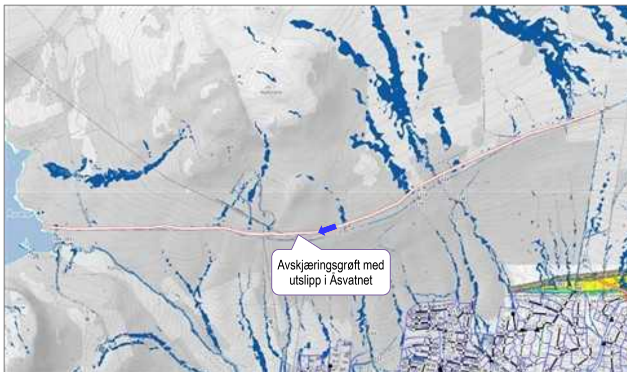
Figur 9.52 Avskjæringsgrøft nord alternativ 2, langs skogsveien på traséen av vannledningen, utslipp i Åsvatnet (vanndybde scenario A 2.2).
