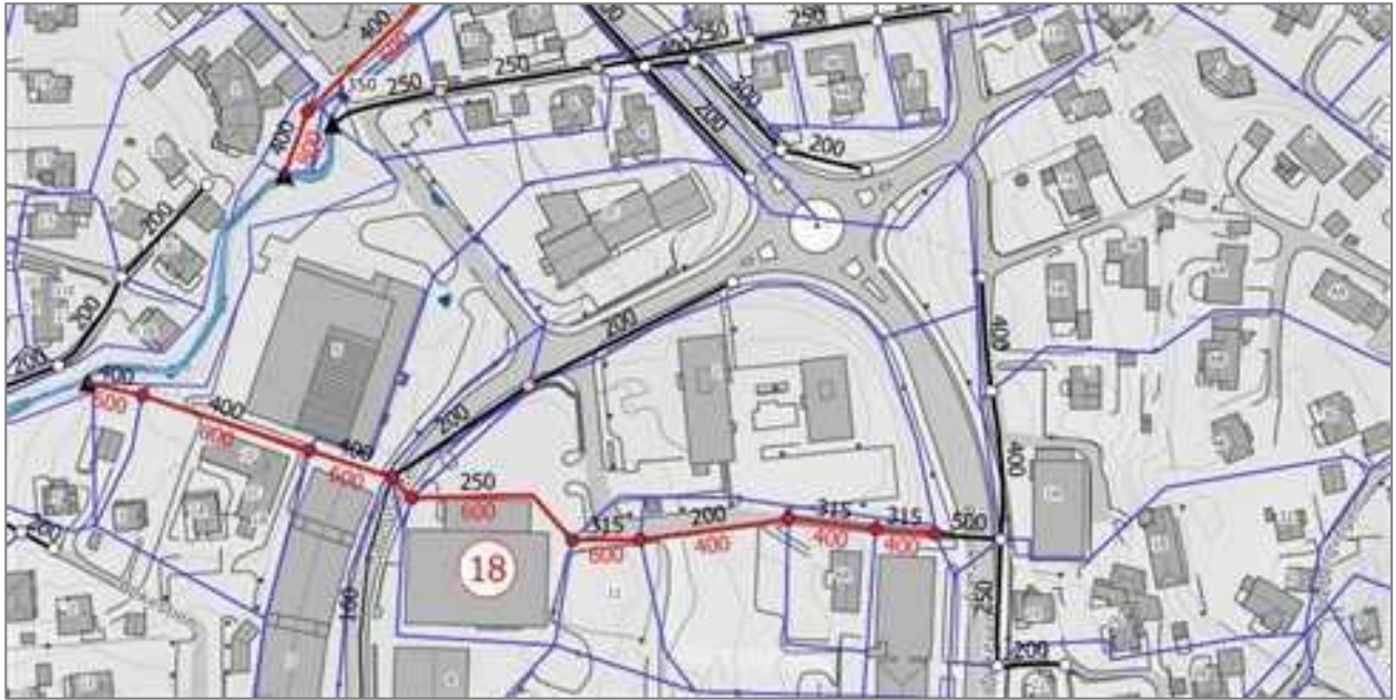
Figur 9.21 Tiltak i ledningsnettets på sted 18 i Jørpeland sentrum, alternativ B (vanndybde scenario A 1.1).
