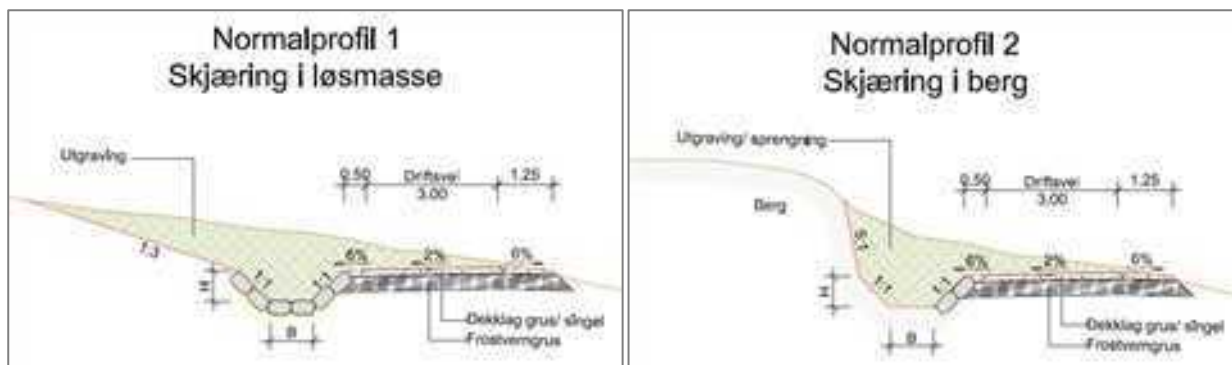
Figur 9.54 Prinsipp tegninger for avskjæringsgrøft og driftsvei ved skjæring i henholdsvis løsmasser (venstre) og berg (høyre).
