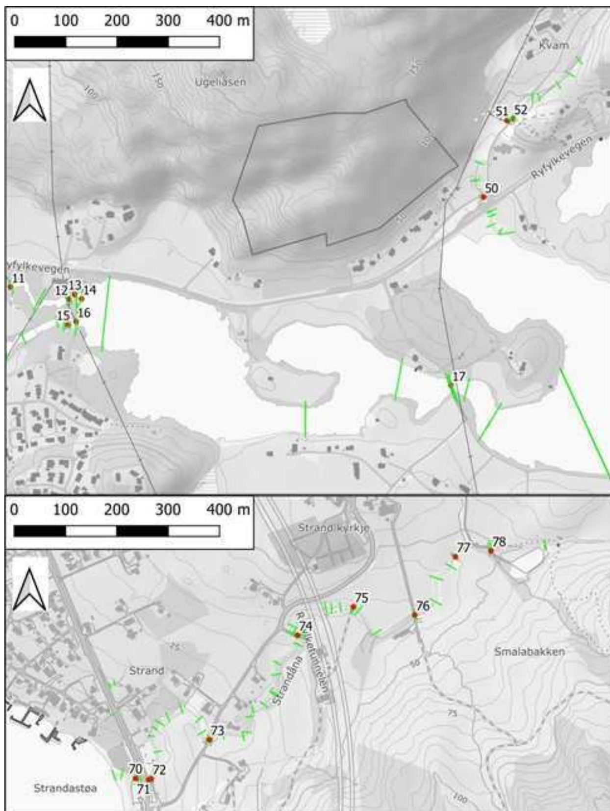
Figur 2 Tverrprofiler og byggverk i Taelva og bekken gjennom Kvam (øverst) og i Strandåna (nederst).
