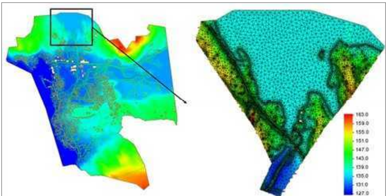
Figur 5.4 Hydraulisk modell for delområdet Tau med utklipp av beregningsnettets rundt utløpet av Nordvatnet. Fargeskalaen viser terrenghøyder i moh +100 m.
