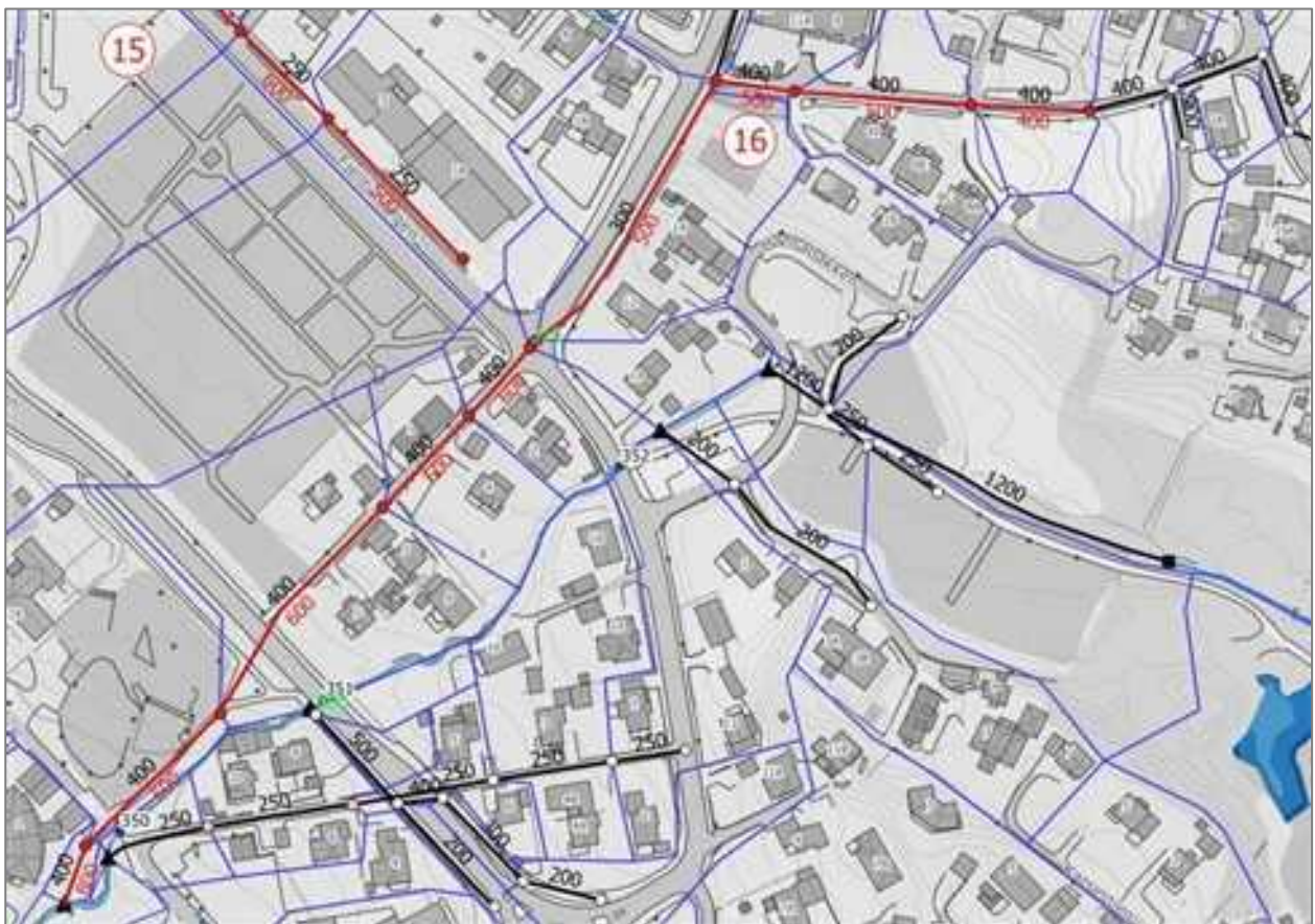
Figur 9.17 Tiltak i ledningsnettets på sted 16 sentralt i Jørpeland, alternativ B (vanndybde scenario A 1.1).
