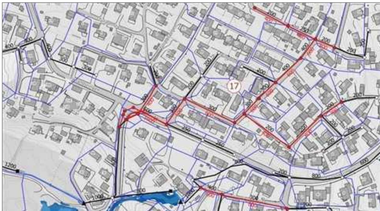
Figur 9.18 Tiltak i ledningsnett på sted 17 sentralt i Jørpeland, alternativ A (vanndybde scenario A 1.1).
