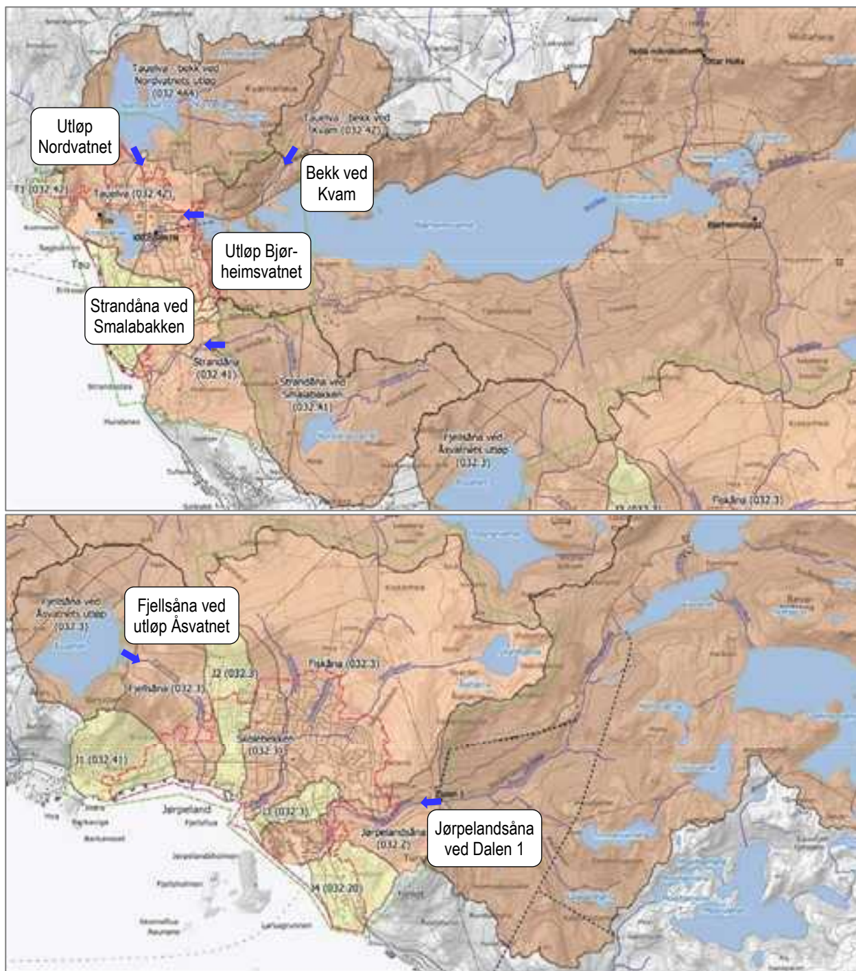
Figur 9.1 Steder ved overgang til hydraulisk modell med beregnet flomvannføring ved hjelp av nedbør-avløps-modell, Tau (øverst) og Jørpeland (nederst).
