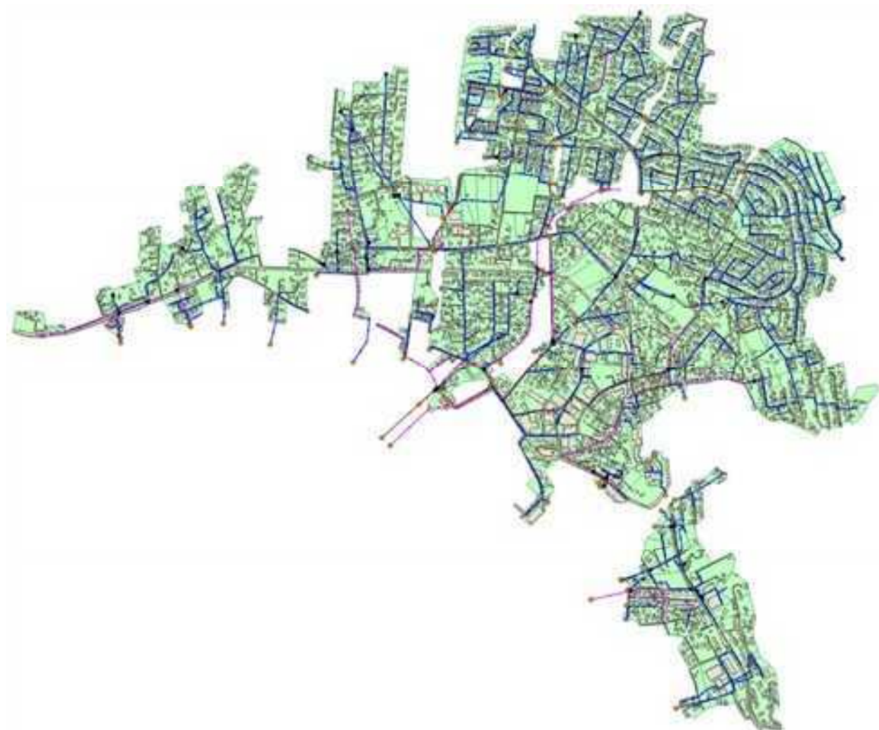
Figur 7.2 Oversikt over ledningsnettmodellen for Jørpeland. Overvannsledninger (blå), avløp felles ledninger (fiolett), spillvannsledninger (brun), utløp (gule prikker) og nedbørfelt til ledningsnettet delt inn etter permeable flater (grønn) og tette flater (rød skravur).
