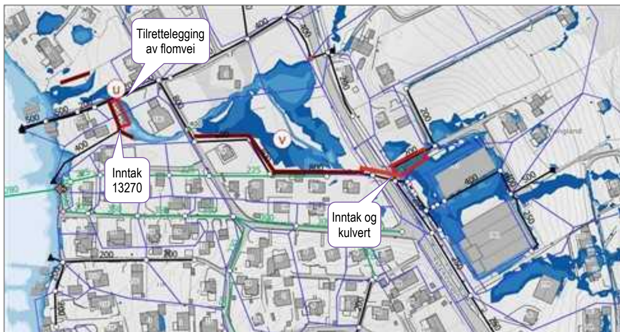
Figur 9.41 Sikring mot 200-års overvannsflom på sted u og v sør i Jørpeland (vanndybde scenario A 2.2).
