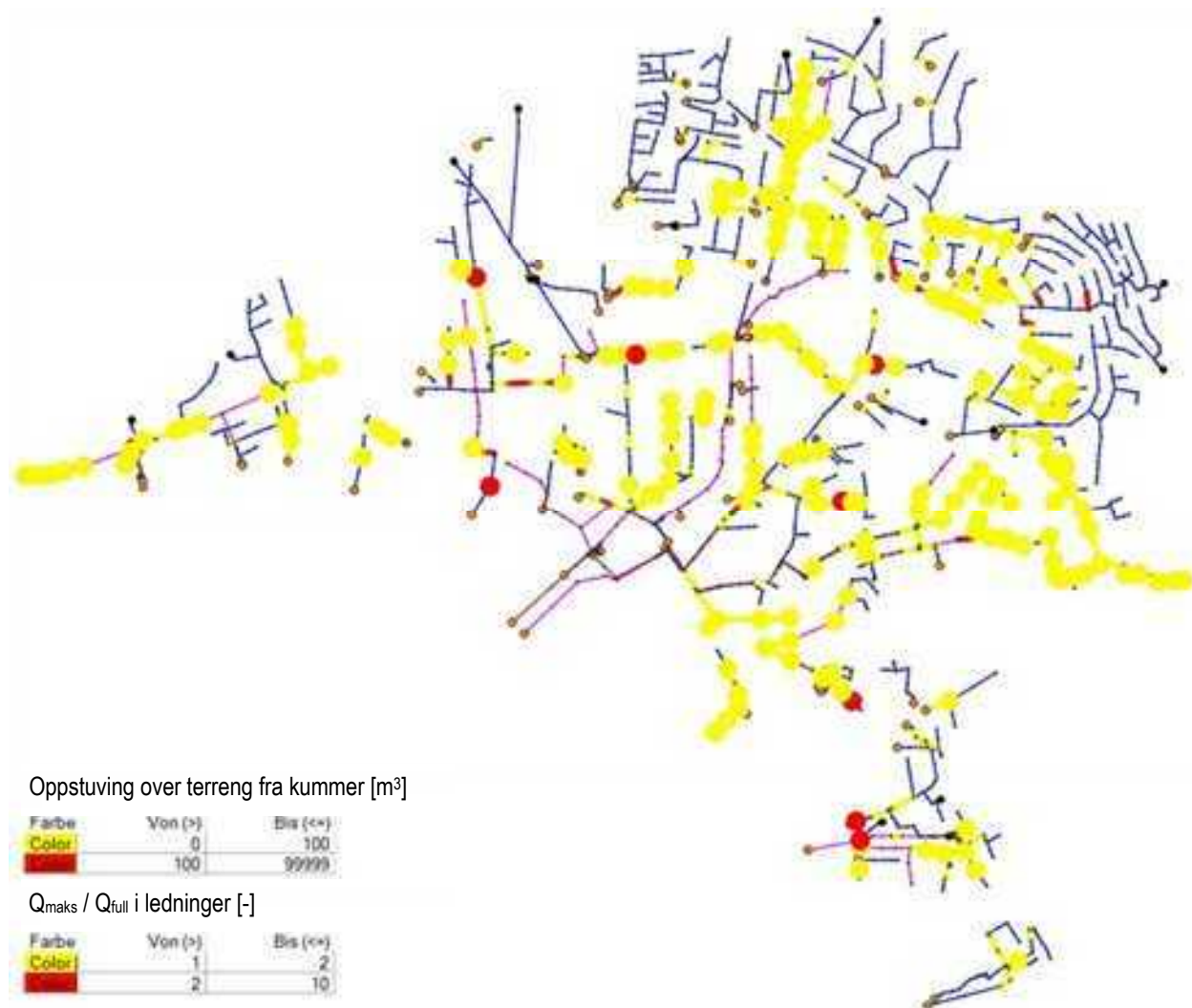
Figur 9.2 Resultater fra koblet ledningsnettberegning Jørpeland scenario A 1.1 (20-års overvannsflom, 10 minutters varighet): Kummer med oppstuvning over terreng og ledninger uten tilstrekkelig kapasitet.
