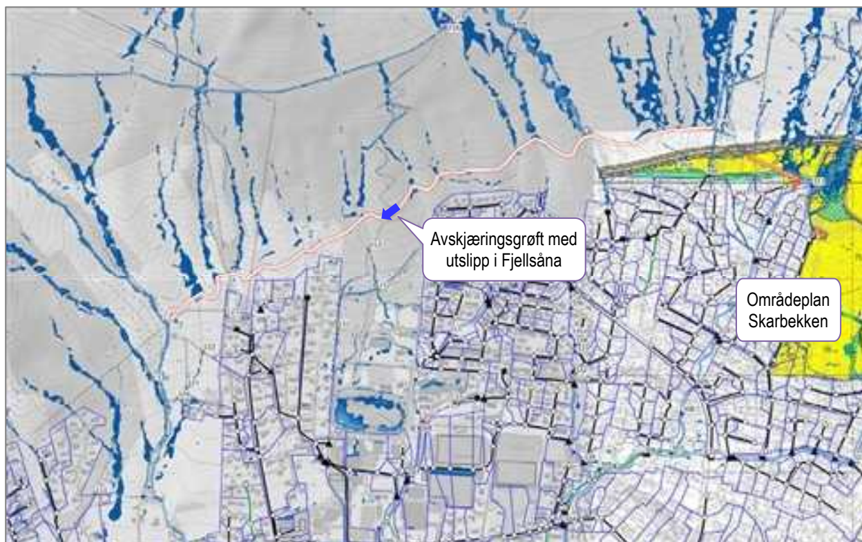
Figur 9.51 Avskjæringsgrøft nord alternativ 1, fra ovenfor boligfeltet Klovsteinen til Fjidlebakke, utslipp i Fjellsåna (vanndybde scenario A 2.2).
