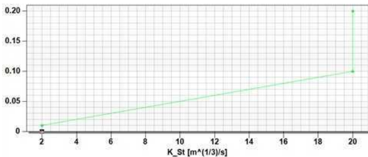
Figur 6.1 Eksempel for dybdeavhengig ruhet. Vanndybde i meter vises på y-aksen, ruhetskoeffisient på x-aksen. For vanndybde \geq 0,1 m er ruhetskoeffisienten konstant.
