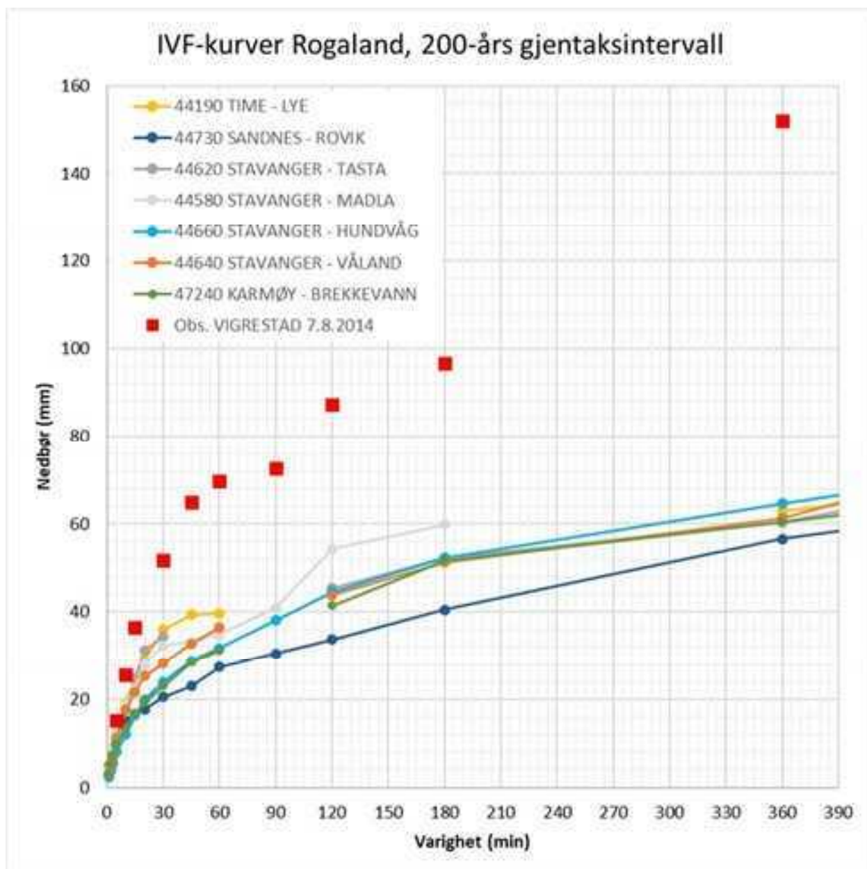
Figur 4.2 IVF-kurver fra nedbørstasjoner i nærheten av Strand kommune for 200-års gjentakintervall; kilde: Klimaservicesenter.no, data til og med år 2020. De røde prikkene viser observerte verdier fra en nedbørhendelse i Vigrestad.
