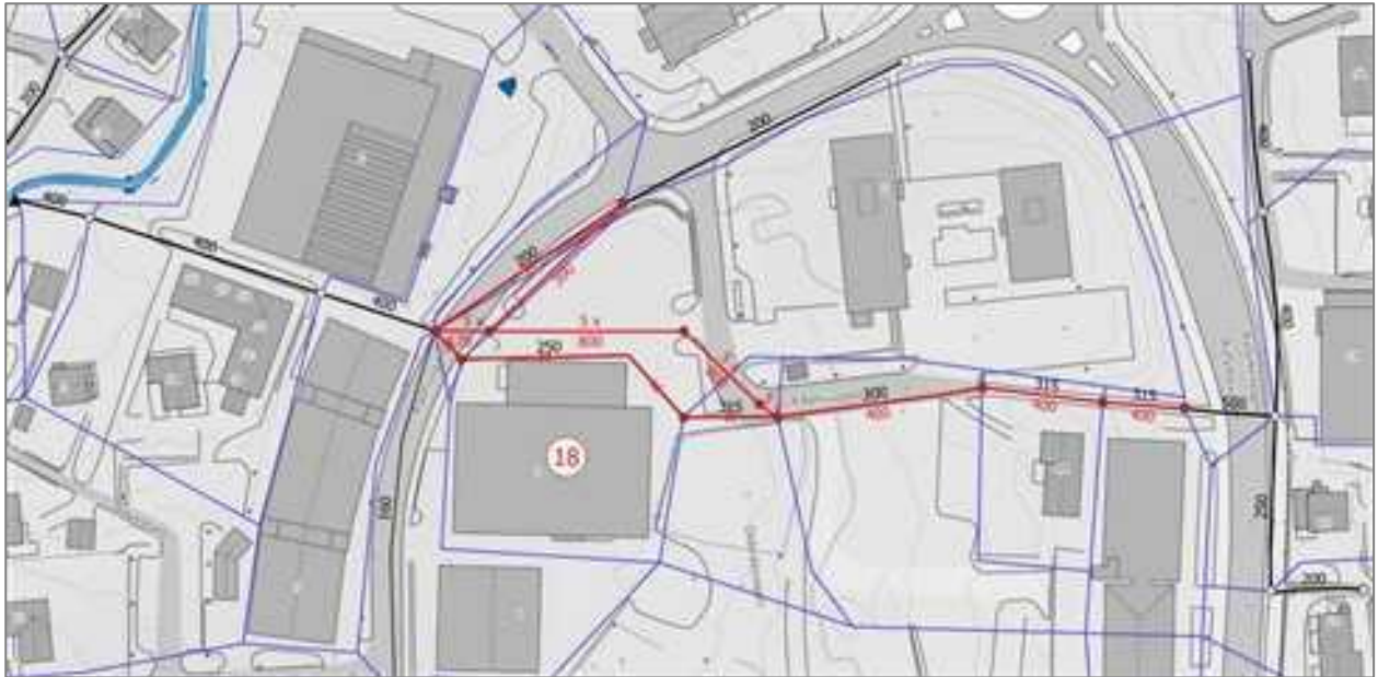
Figur 9.20 Tiltak i ledningsnettets på sted 18 i Jørpeland sentrum, alternativ A (vanndybde scenario A 1.1).
