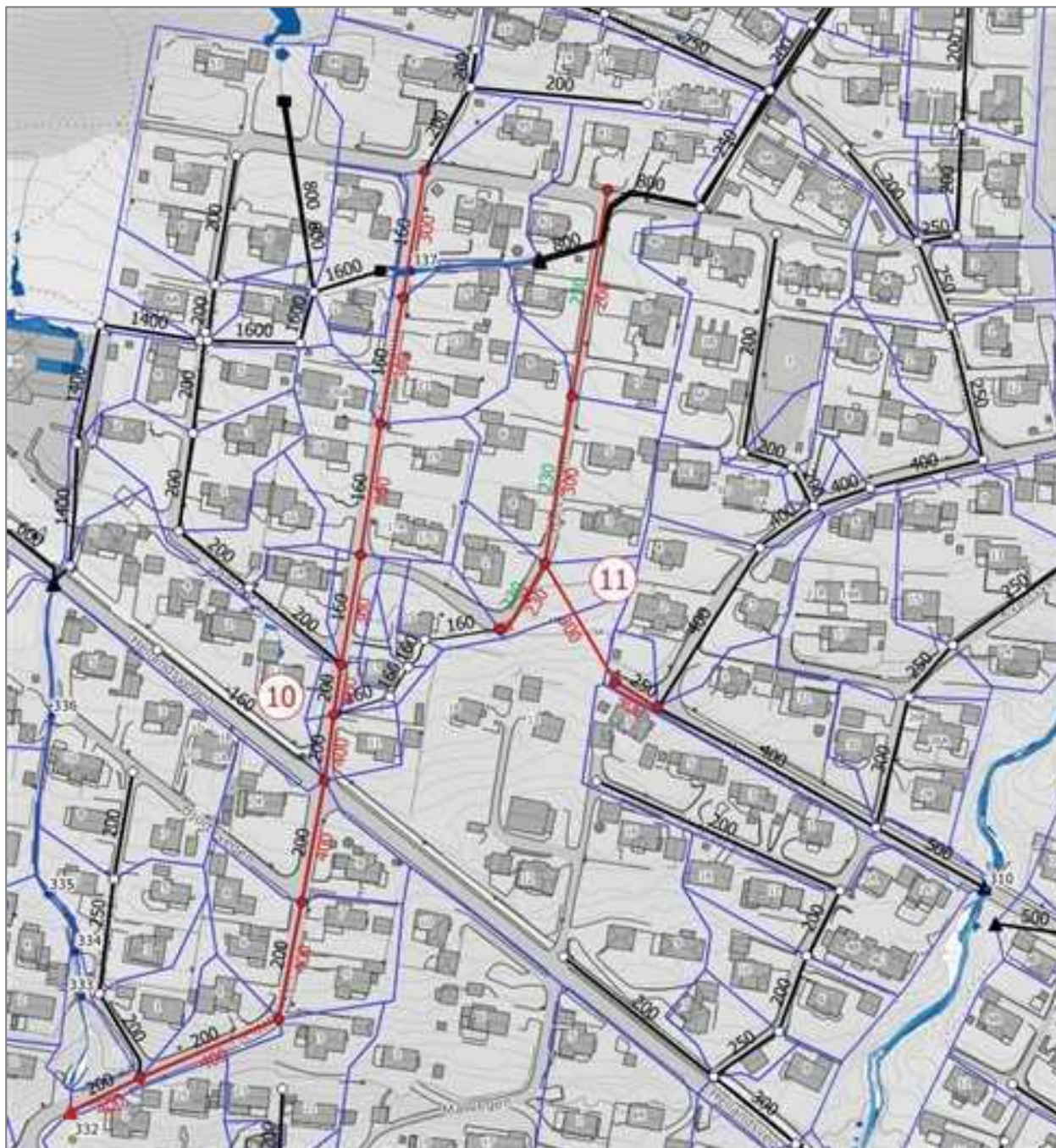
Figur 9.13 Tiltak i ledningsnettets på sted 10 og 11 nord i Jørpeland (vanndybde scenario A 1.1).
