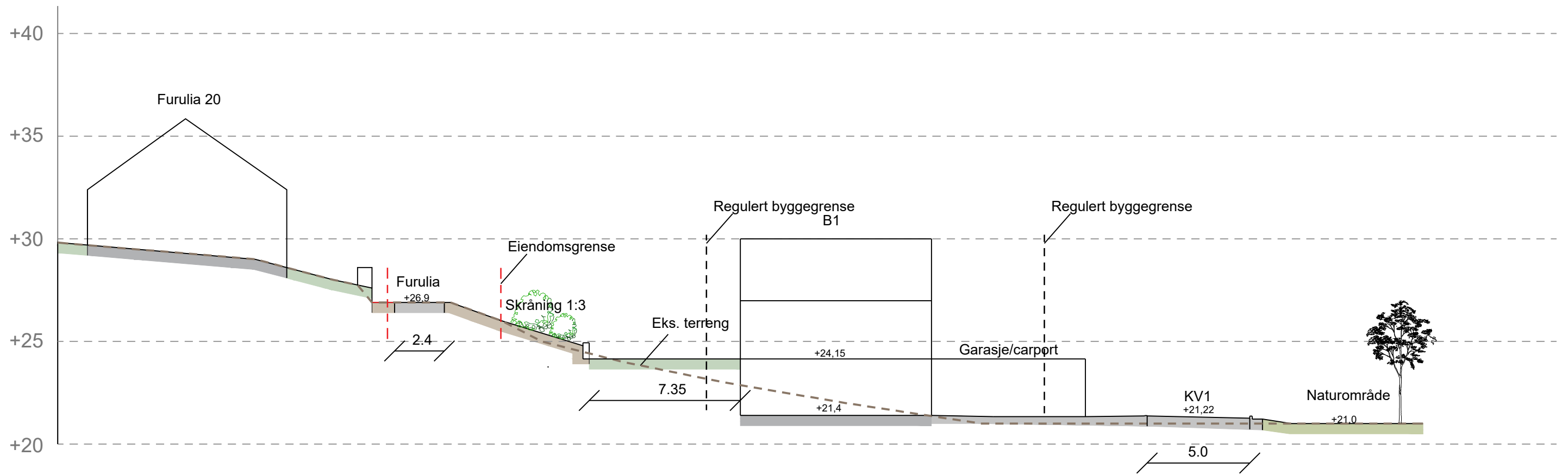
Snitt AA'
