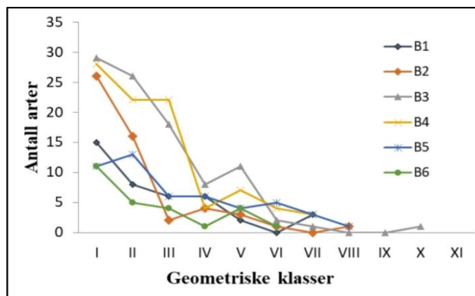
Figur 42. Faunastruktur uttrykt i geometriske klasser for stasjonene B1-B6 tatt under Marin Overvåking Rogaland, 11.-13. juli 2017. Antall arter langs y – akse og geometriske klasser langs x-aksen.
