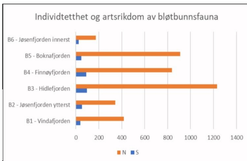
Figur 59. Sammenligning av individtetthet ( N ) og artsrikdom ( S ) på de seks stasjonene i Boknafjord-systemet undersøkt ved Marin Overvåking Rogaland i juli 2017.
