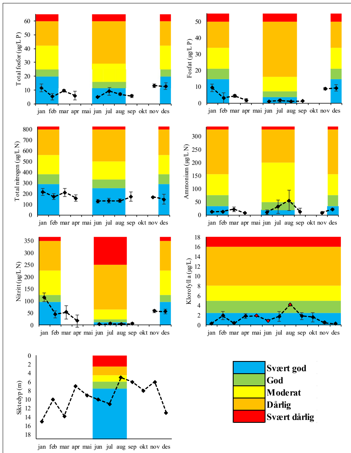
Figur 13. Linjediagram med gjennomsnittlig innhold av total fosfor ( \mu\text{g/L} ), fosfat ( \mu\text{g/L} ), totalt nitrogen ( \mu\text{g/L} ), ammonium ( \mu\text{g/L} ), nitrat ( \mu\text{g/L} ), klorofyll a ( \mu\text{g/L} ) og siktedyb (m) med standardavvik i vannsøylen i Krossfjorden (C) i 2017. Tilstandsklasser er markert med farge etter veileder 02:2013.
