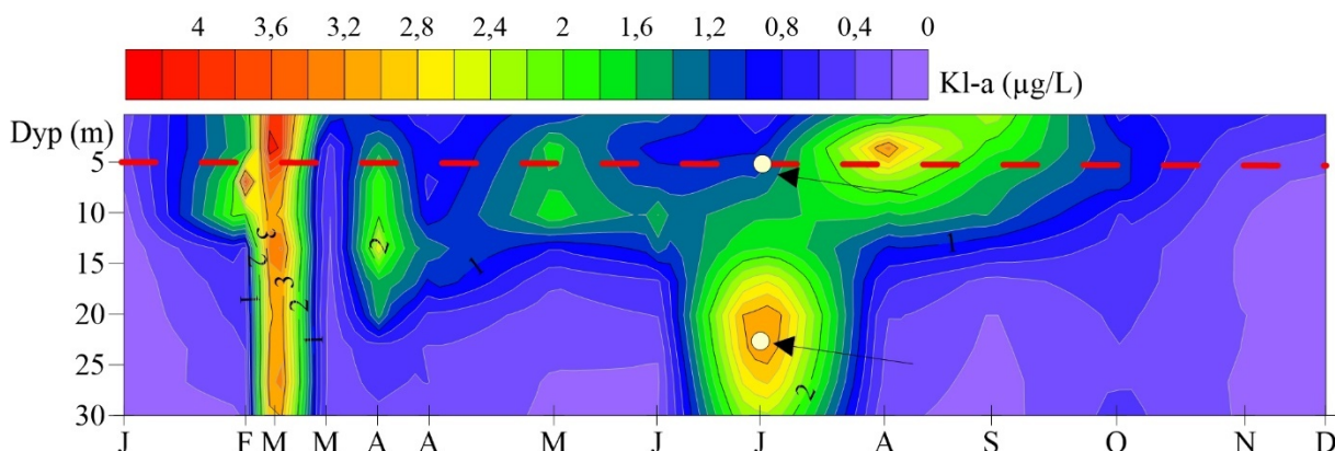
Figur 58. Konturplott av klorofyll- a ( \mu\text{g/L} ) i vannsøylen i Jelsaffjorden (J). Y akse viser dybder fra 0-30 m og x akse viser til tidspunkt for prøvetaking. Fargeskalaen er relativ, med lilla for de laveste verdiene og rød for de høyeste. Stiplet rød linje indikerer 5 m dyp for prøvetaking av klorofyll- a prøver. Sirkler ved juli illustrerer ulik algebiomasse ved ulike dyp for juli måned.
