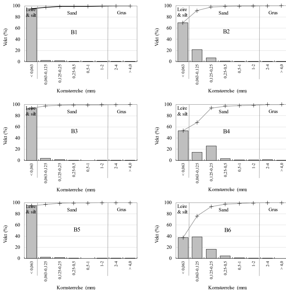
Figur 41. Kornfordeling for stasjon B1-B6. Figuren viser kornstørrelse langs x-aksen og henholdsvis akkumulert vektprosent og andel i hver størrelseskategori langs y-aksen.
