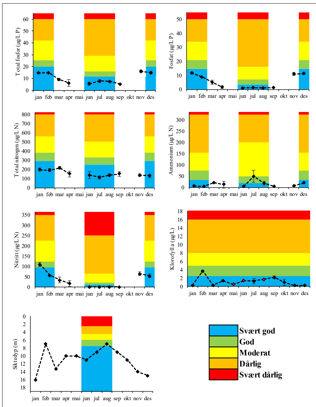
Figur 22. Linjediagram med gjennomsnittlig innhold av total fosfor ( \mu\text{g/L} ), fosfat ( \mu\text{g/L} ), totalt nitrogen ( \mu\text{g/L} ), ammonium ( \mu\text{g/L} ), nitrat ( \mu\text{g/L} ), klorofyll a ( \mu\text{g/L} ) og siktedyp (m) med standardavvik i vannsøylen for Hidleffjorden (F) i 2017. Tilstandsklasser er markert med farge etter veileder 02:2013..
