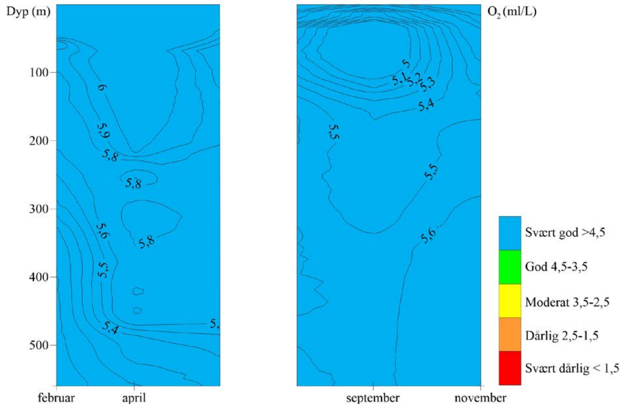
Figur 36. Konturplott av oksygeninnhold (ml/L O_2 ) i Boknafjorden (K). Y akse viser dybder fra 0-559 m og x akse viser til tidspunkt for prøvetaking. Fargeskalaen er basert på grenseverdier fra veileder 02:2013. Hvitt felt i grafen markerer at det ikke ble tatt prøver fra april til september.
