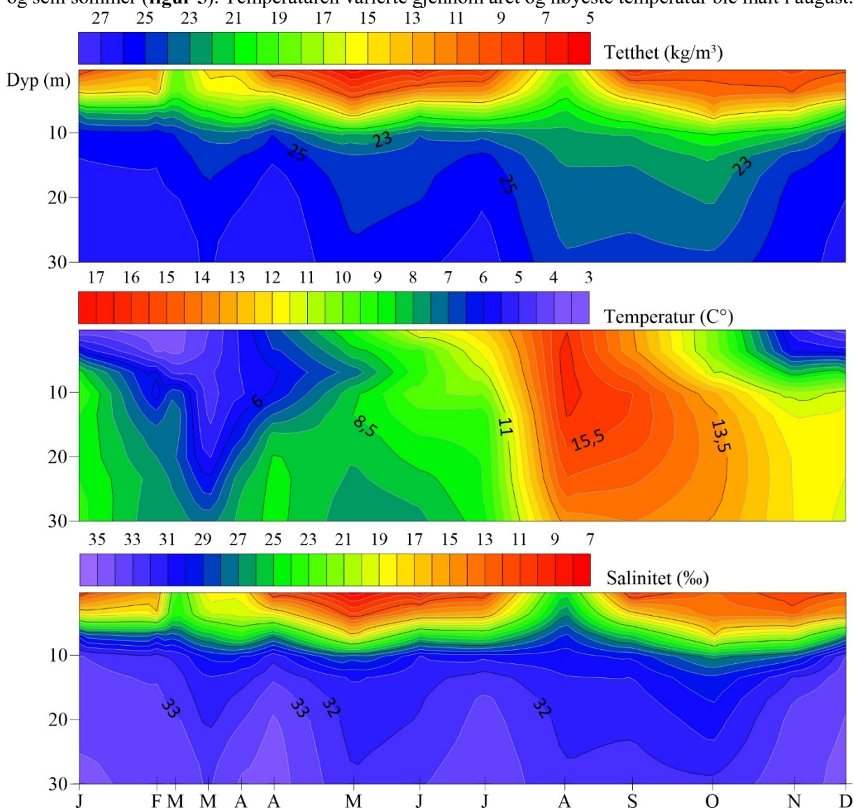
Figur 5. Konturplott av tetthet, temperatur (°C) og salinitet (‰) i vannsøylen i Sandsfjorden (A). Y akse viser dybder fra 0-30 m og x akse viser til tidspunkt for prøvetaking (f. eks. J=januar). Fargeskalaen er relativ, med lilla for de laveste verdiene og rød for de høyeste for temperatur og motsatt for tetthet og salinitet.
