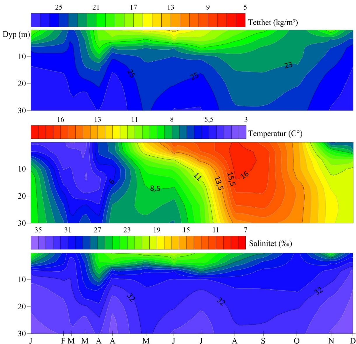
Figur 38. Konturplott av tetthet, temperatur (°C) og salinitet (‰) i vannsøylen på stasjon Jøsefjorden indre (L). Y-akse viser dybder fra 0-30 m og x-akse viser til tidspunkt for prøvetaking. Fargeskalaen er relativ, med lilla for de laveste verdiene og rød for de høyeste for temperatur og motsatt for tetthet og salinitet.
