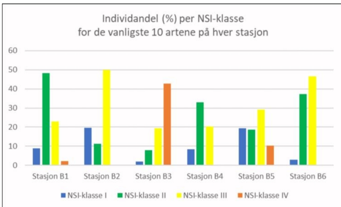
Figur 60. Relativ dominans av arter som er sensitive (NSI-klasse I) til tolerante (NSI-klasse IV) overfor organiske tilførsler blant de ti mest vanlige artene på stasjon B1-B6 under Marin Overvåking Rogaland i sommer 2017, presentert som andel (%) av den totale faunaen på hver stasjon.
