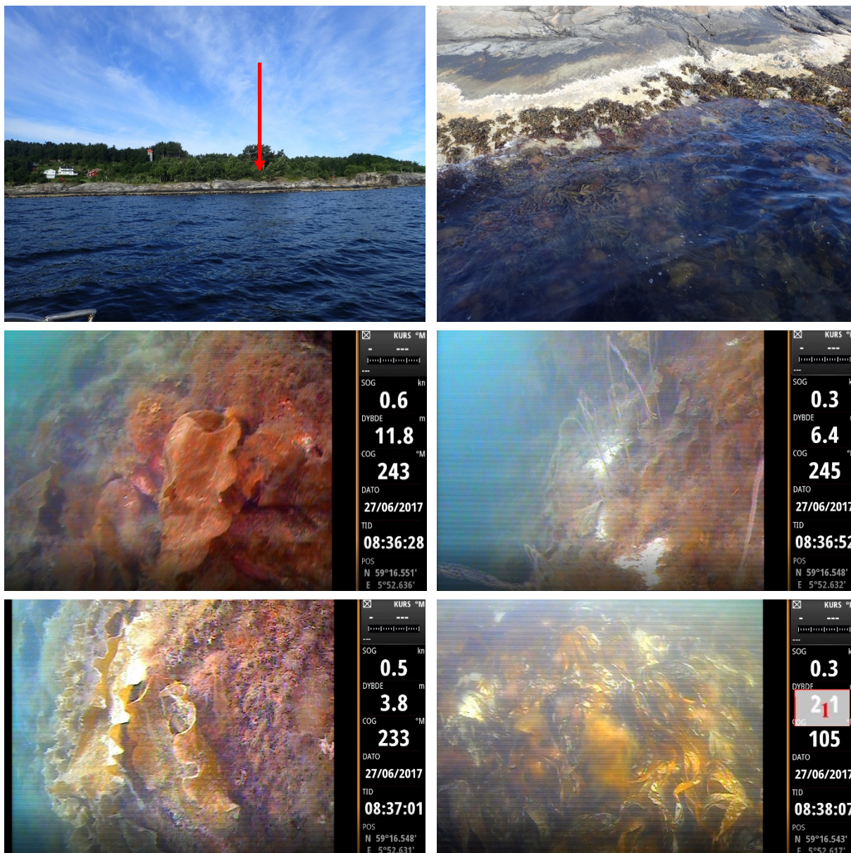
Figur 51. St. 19 Bjergøy Øverst t.h.: Oversikt over Bjergøy med rød pil som viser til slutt punkt for transektet. Øverst t.v.: Oversiktsbilde av fjæresonen ved slutt punkt. Midten: Hardbunn ved 12-11 m med spredt sukkertare (t.v.) og 6 m dyp på sandbunn med algematter og spredt vekst av sukkertare (t.h.). Nederst: Fjell på 3-4 m dyp med sukkertare og små alger (t.v.) fingertare på 0,5 m dyp (t.h.).
