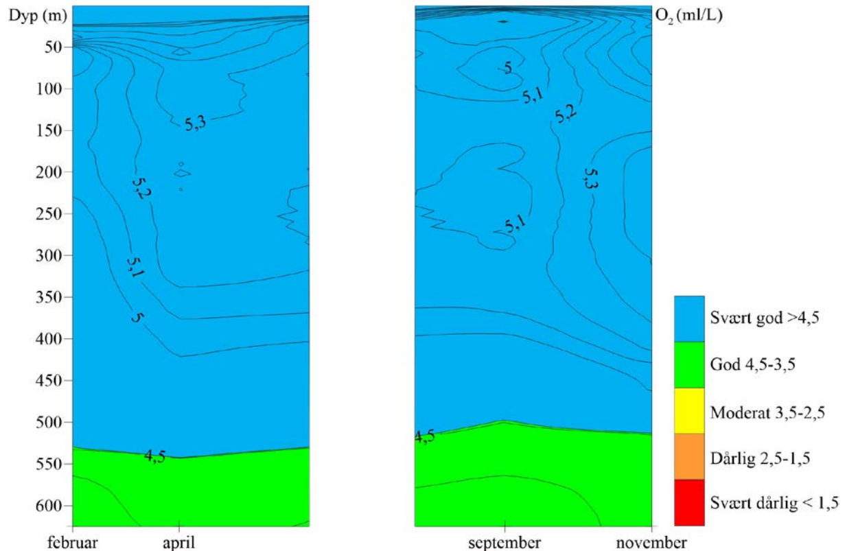
Figur 9. Konturplott av oksygeninnhold (ml/L O 2 ) i vannsøylen i Vindafjorden (B). Y akse viser dybder fra 0-623 m og x akse viser til tidspunkt for prøvetaking. Fargeskalaen er basert på grenseverdier fra veileder 02:2013. Hvitt felt i grafen markerer at det ikke ble tatt prøver fra april til september.
