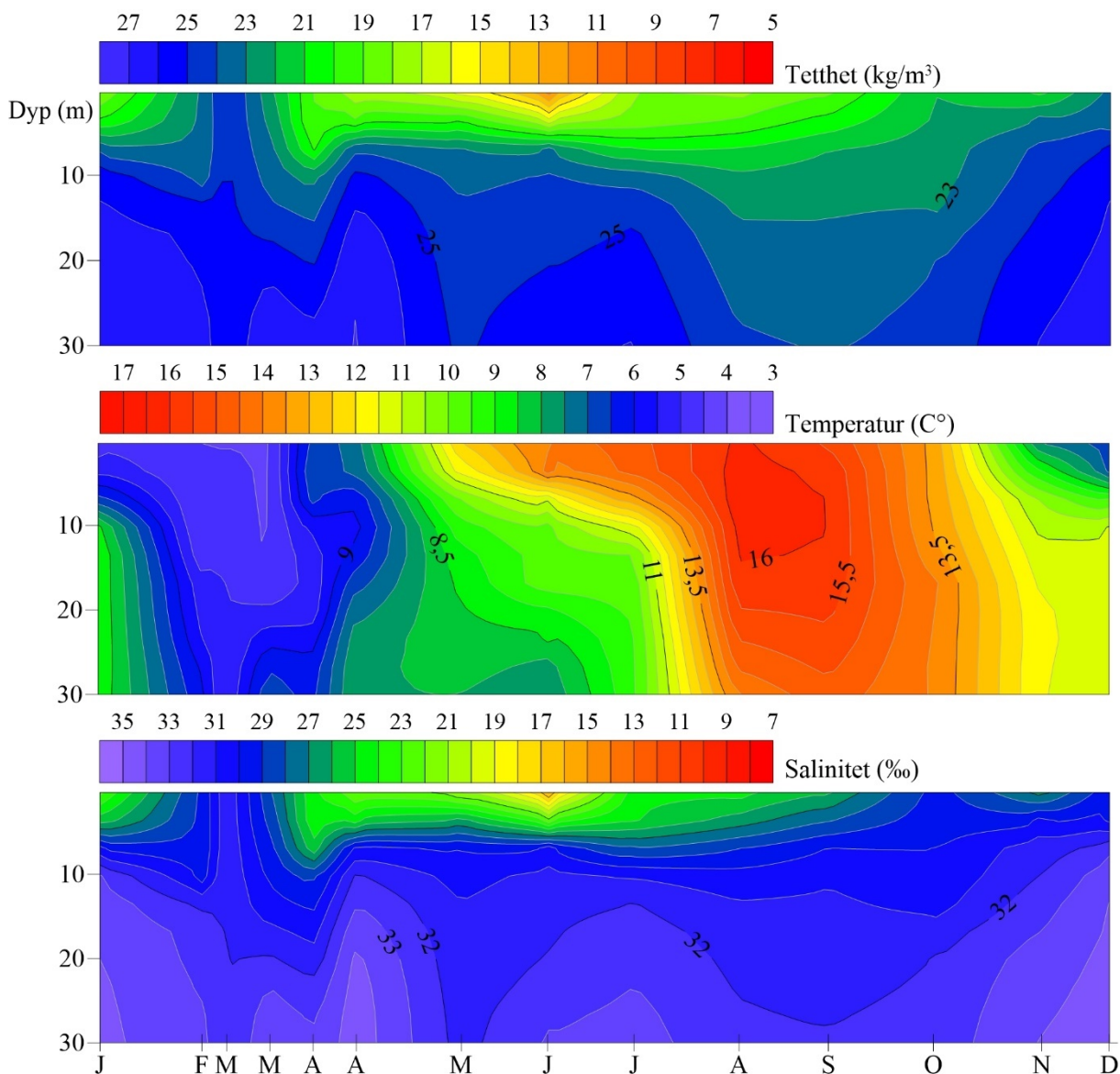
Figur 17. Konturplott av tetthet, temperatur (°C) og salinitet (‰) i vannsøylen i Jøsefjorden ytre. Y akse viser dybder fra 0-30 m og x akse viser til tidspunkt for prøvetaking (f. eks. J=januar). Fargeskalaen er relativ, med lilla for de laveste verdiene og rød for de høyeste for temperatur og motsatt for tetthet og salinitet
