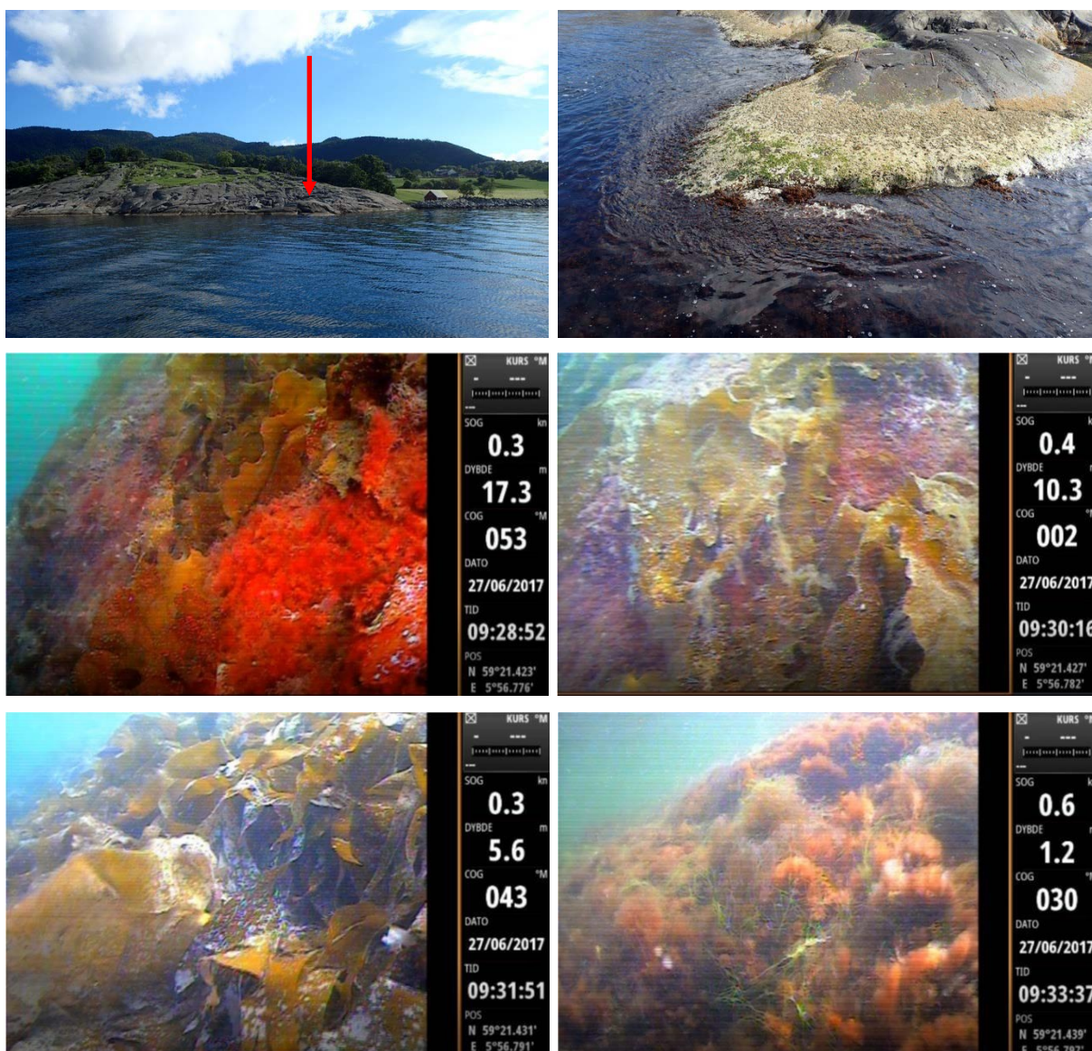
Figur 50. St. 17 Kvernaneset. Øverst t.h: Oversikt over Kvernaneset med rød pil som viser til slutt punkt for transektet. Øverst t.v: Oversiktsbilde av fjæresonen ved slutt punkt. Midten: Hardbunn på 17 m (t.v.) og 10 m dyp med spredt til dominerende sukkertare. Nederst: Tareskog på 5-6 m dyp (t.v.), mosaikk av rødalger og trådformede grønnalger på fjellbunn (t.h.) på 1 m dyp.
