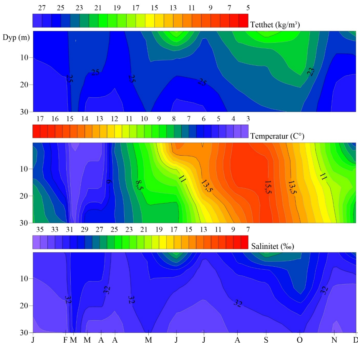
Figur 35. Konturplott av tetthet, temperatur (°C) og salinitet (‰) i vannsøylen i Boknafjorden (K). Y-akse viser dybder fra 0-30 m og x-akse viser til tidspunkt for prøvetaking (f. eks. J=januar). Fargeskalaen er relativ, med lilla for de laveste verdiene og rød for de høyeste for temperatur og motsatt for tetthet og salinitet.
